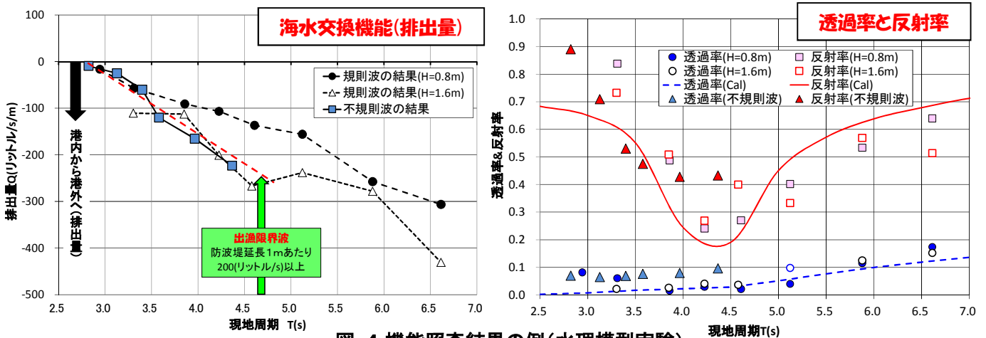
図-4 機能照査結果の例(水理模型実験)
