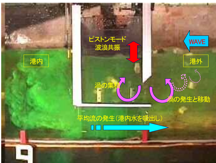
図-2 基本原理モデル図
