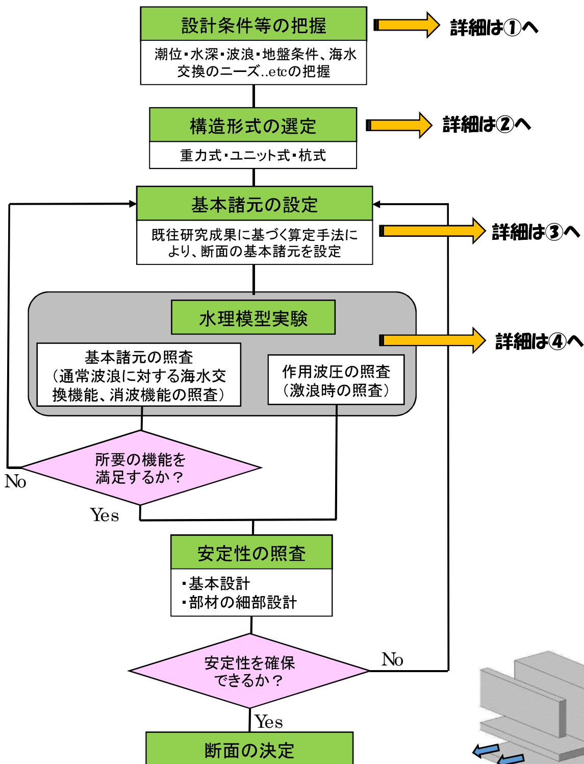
図- 設計フロー
