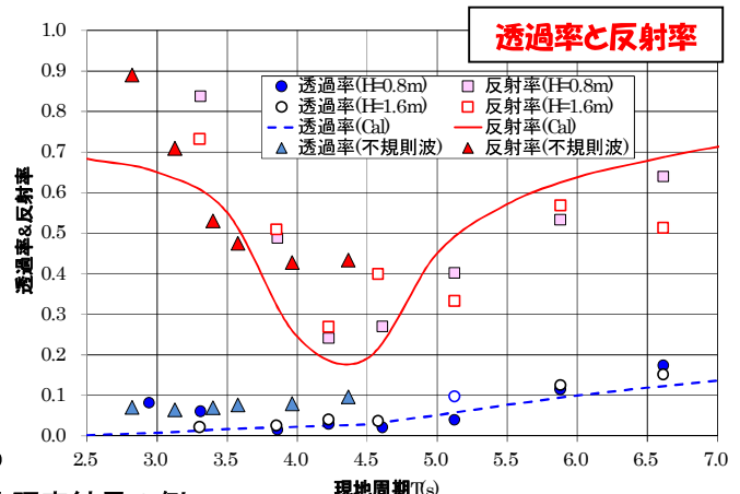
図- 機能照査結果の例
