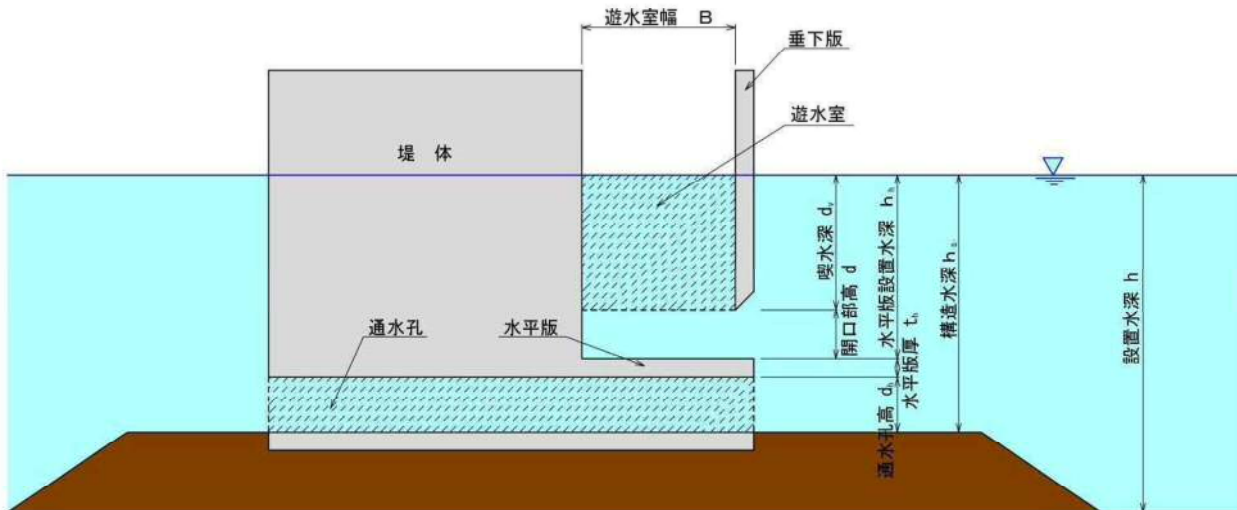
図- 基本断面図
